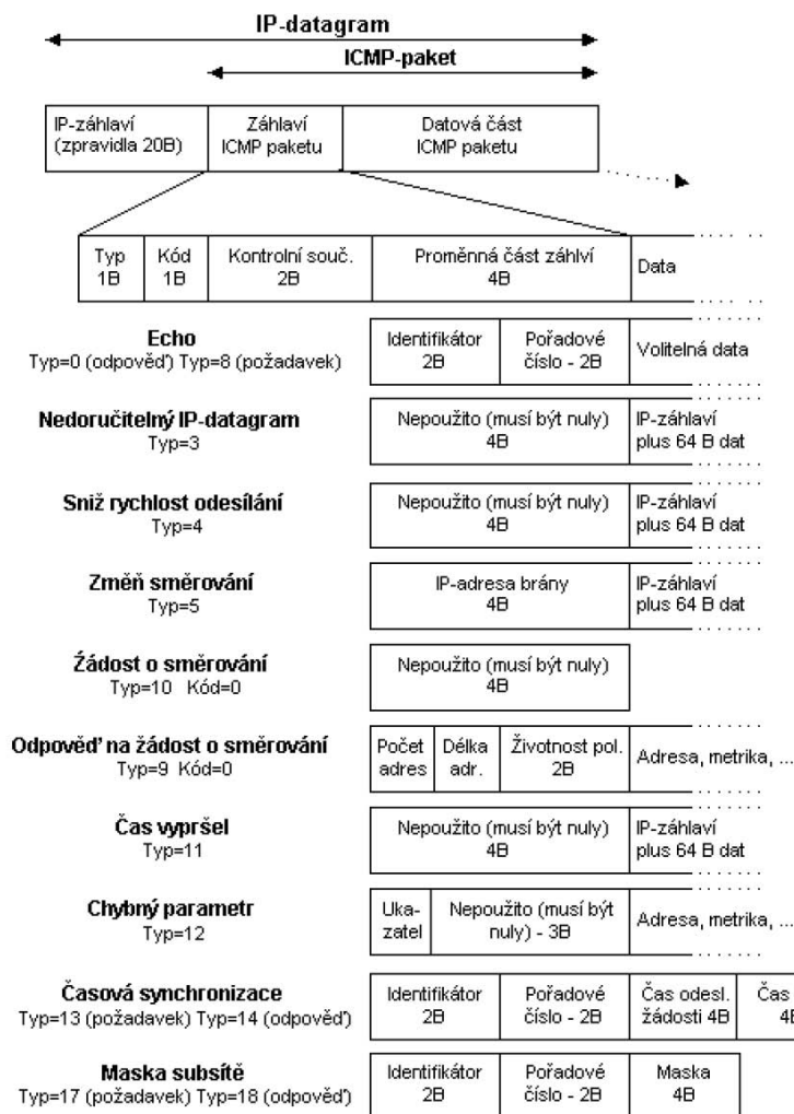
Obr. 5.10 ICMP-paket
